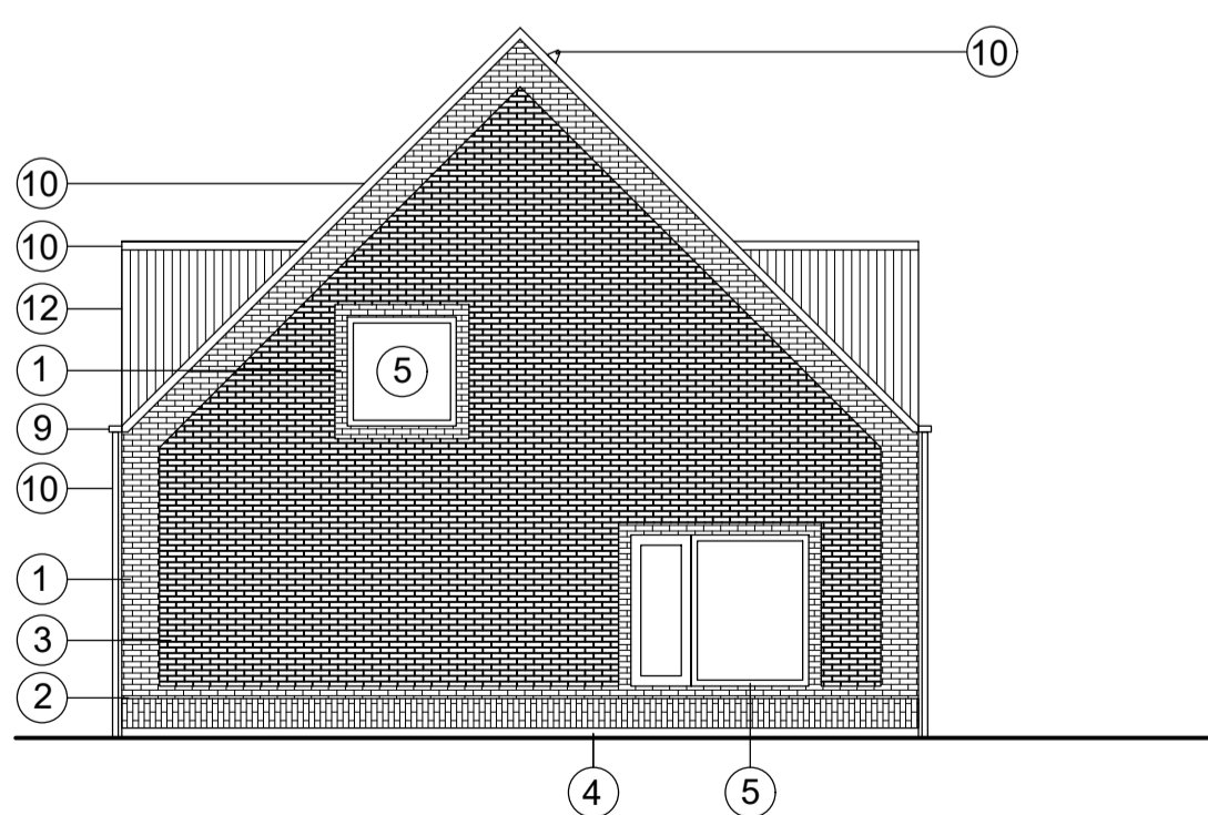
FASAD VÄSTER
