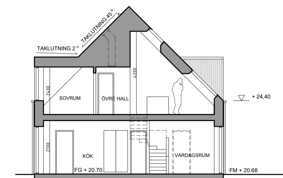
SEKTION A
