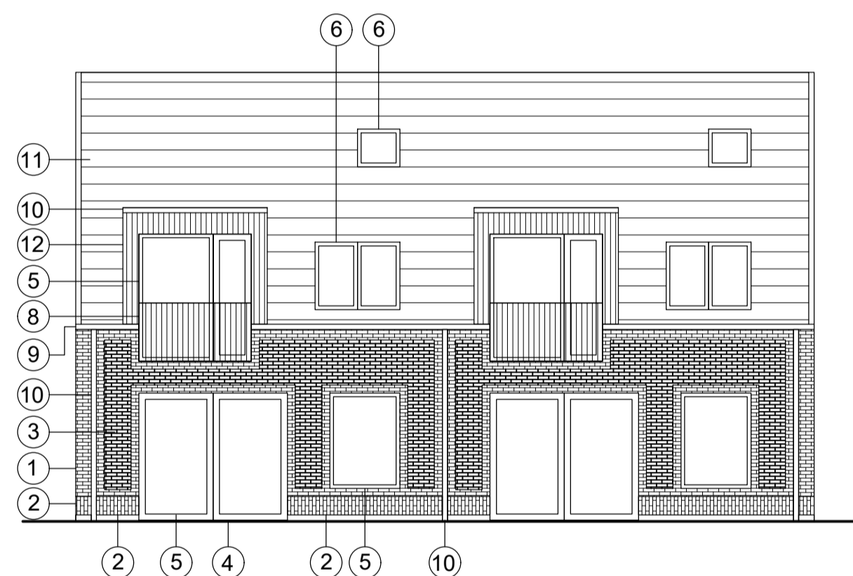
FASAD SÖDER
