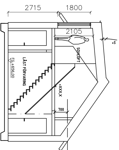
SEKTION B-B SKALA 1:100
