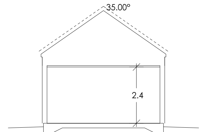
SEKTION A-A
