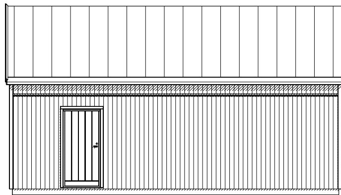
FASAD 4
