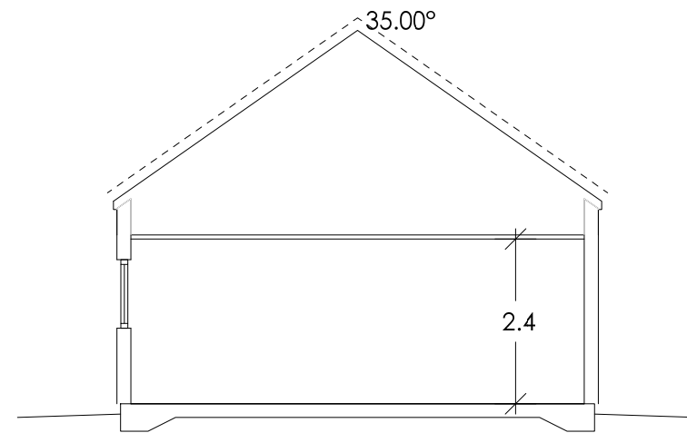
SEKTION A-A
