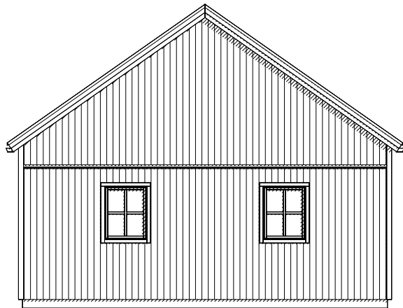
FASAD 3
