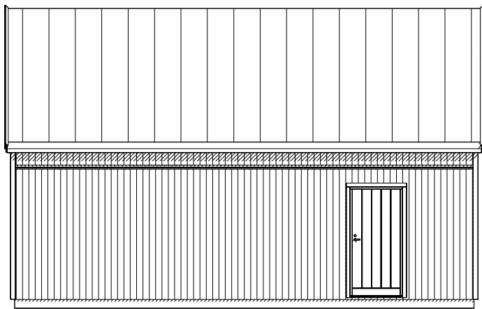
FASAD 2
