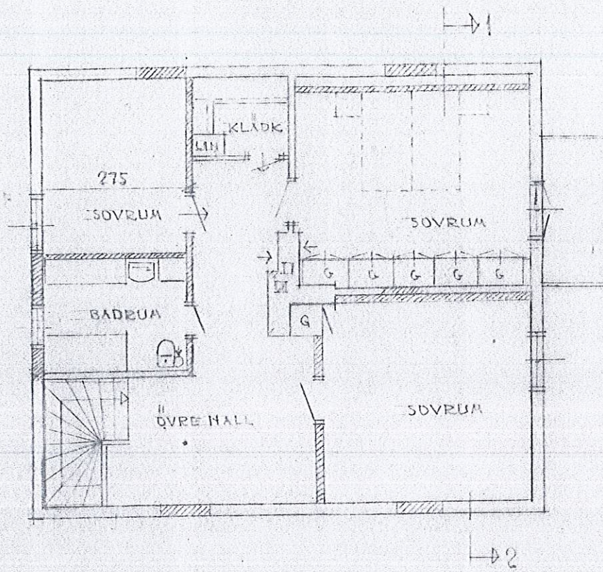
ÖVRE VÄNING
