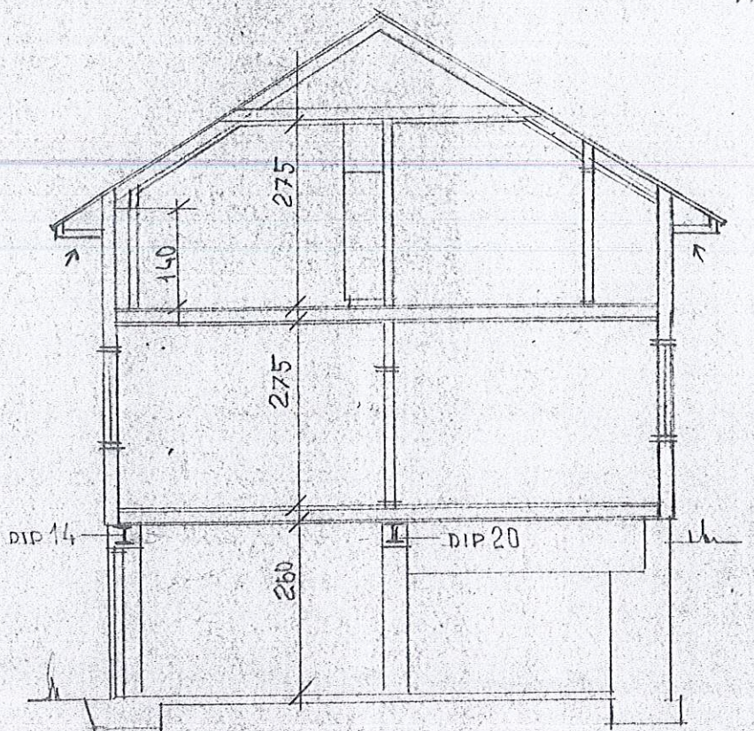
SEKTION
