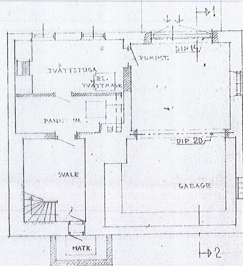
KÄLLARVÄNING
