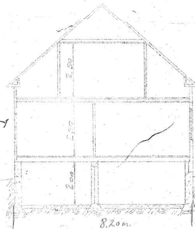
SECTION A-B
