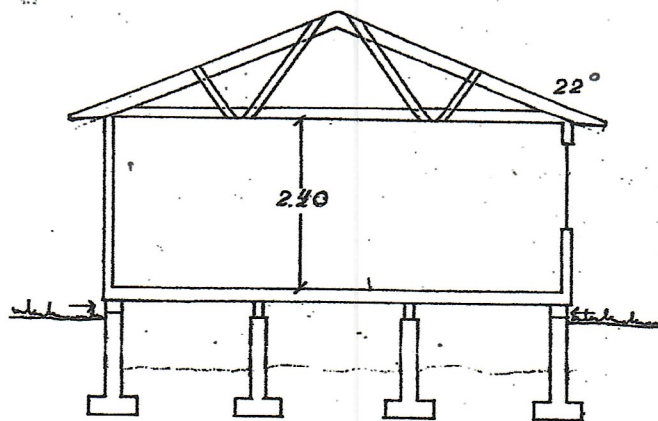
SEKTION
