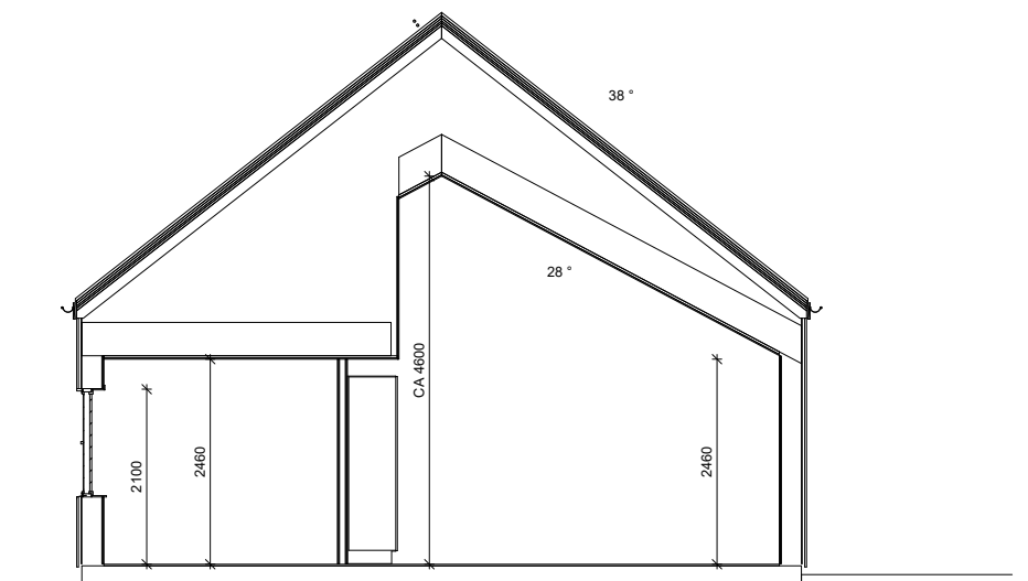
SEKTION B-B
