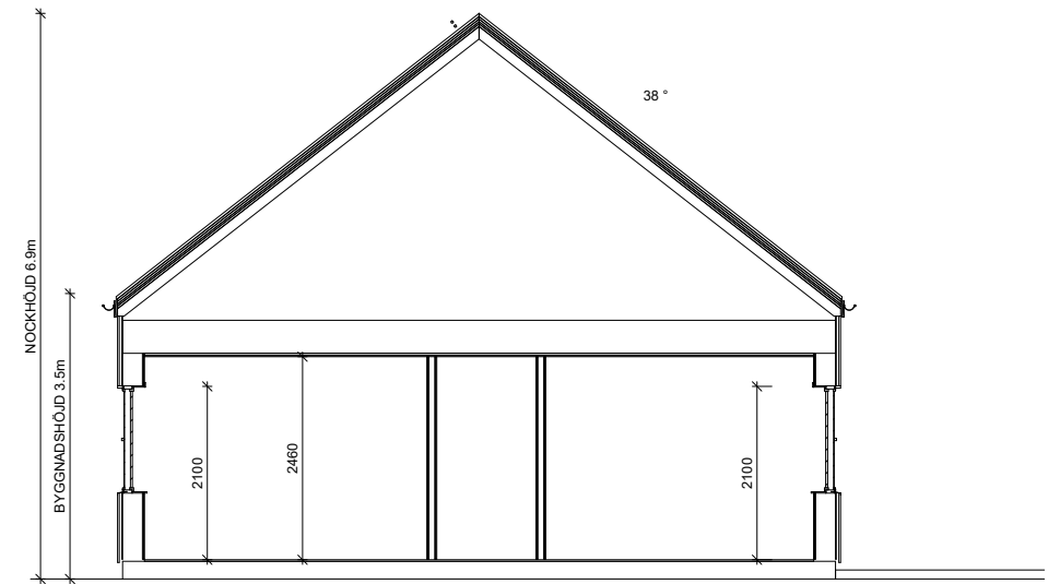
SEKTION A-A
