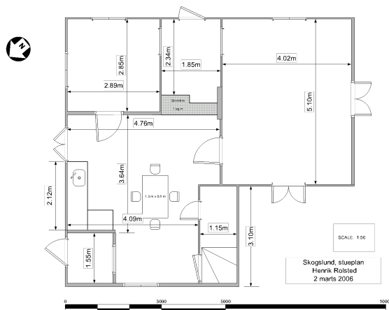
Grundplan efter udvidelse og indretning køkken
