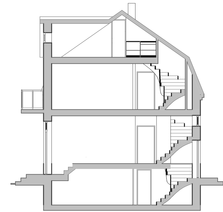
Sektion A-A 1:100
