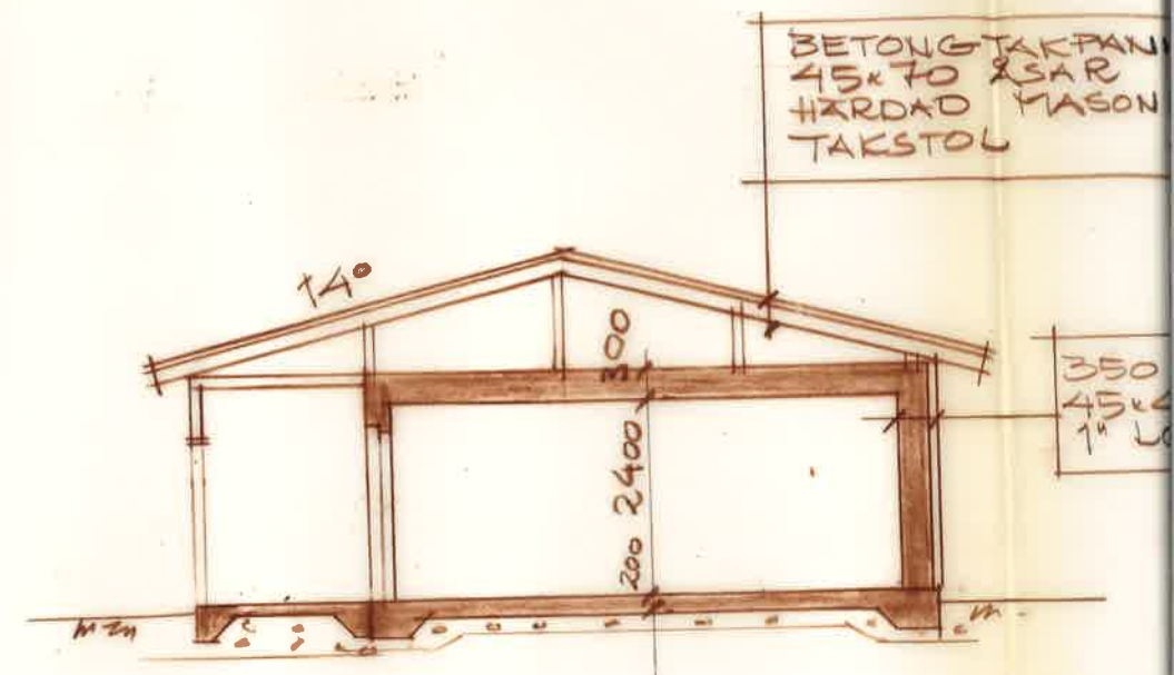
SEKTION 1:100
