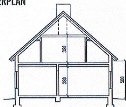
SEKTION
