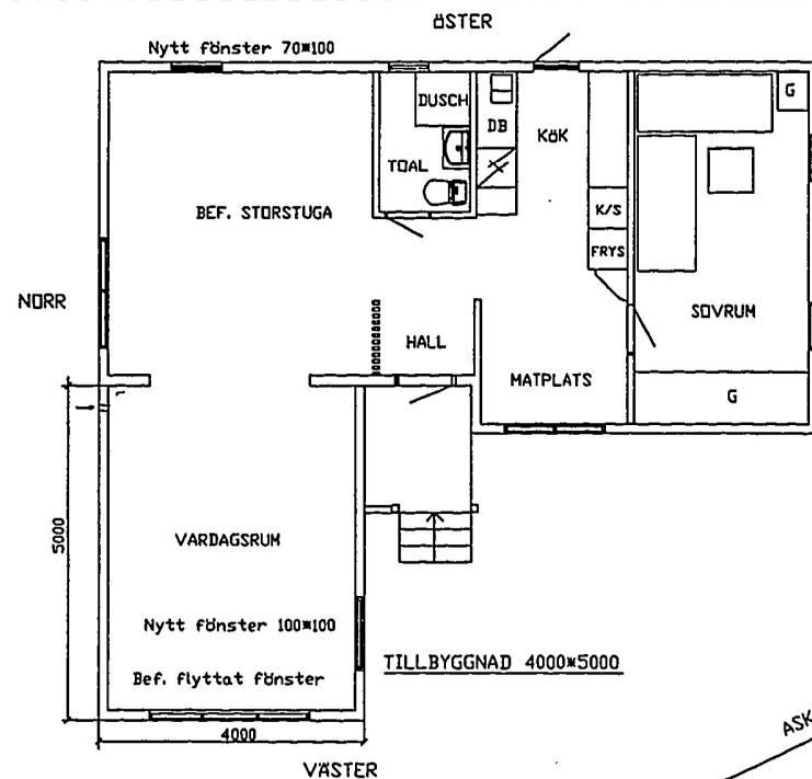
PLAN SKALA 1:100
