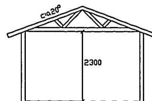
SEKTION SKALA 1:100
