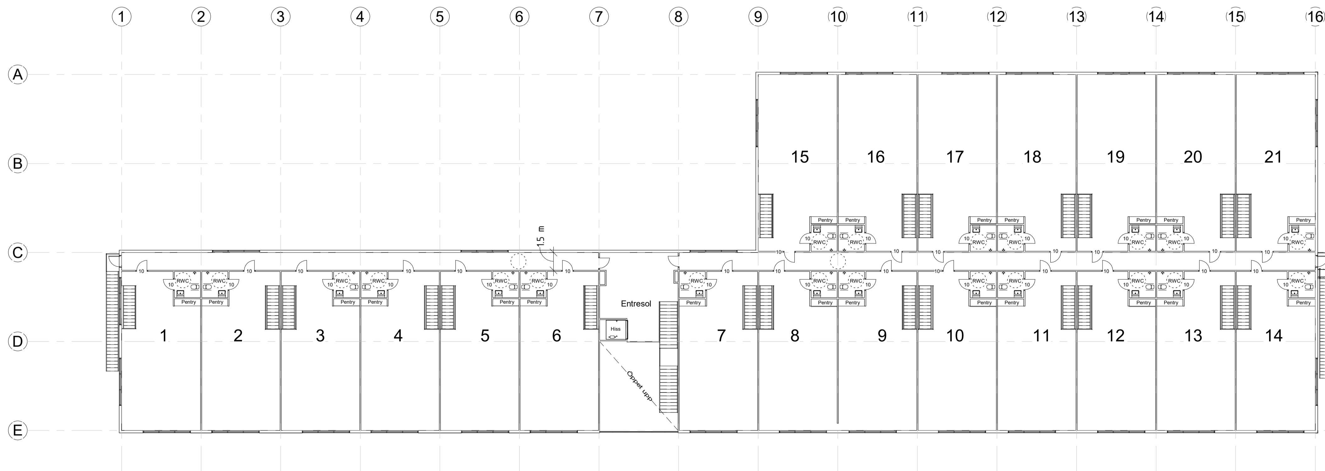
2 Plan 2 1 : 200
