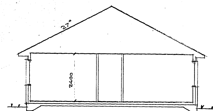
SEKTION
