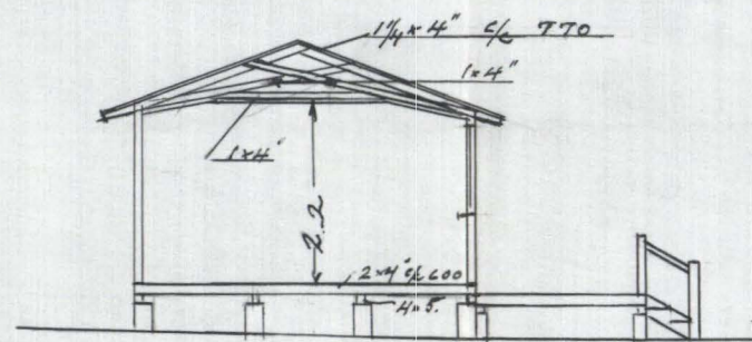
Section A-B
