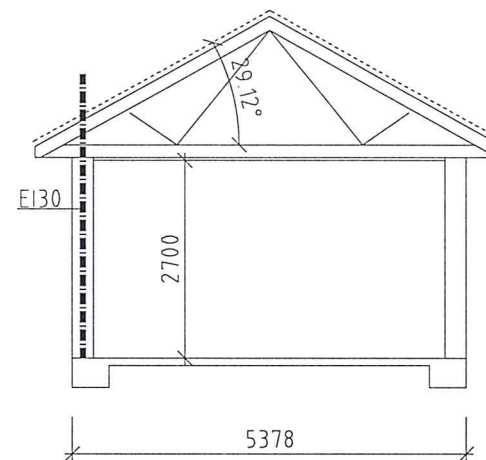
SEKTION B
