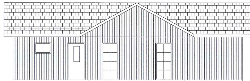
FASAD ÖSTER
