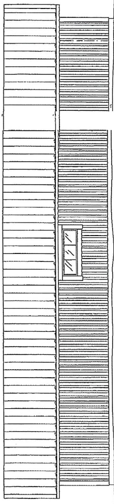
FASADER MOT NORR OCH SÖDER
