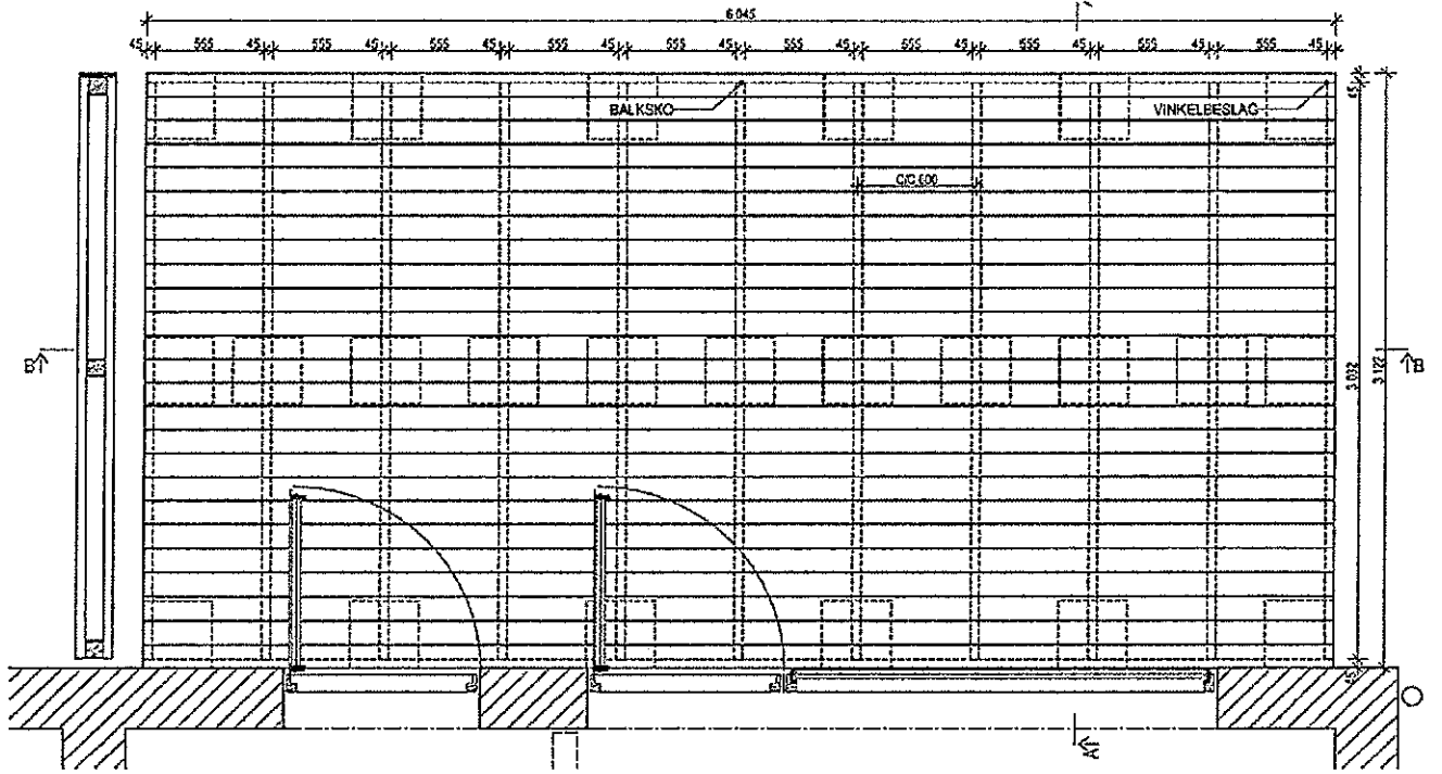
PLAN SKALA 1:20
