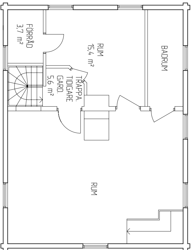
PLAN 2 1:100 BRA: 78,9 m²
